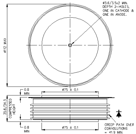
W29 - 100A342
