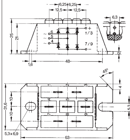
X117b FO-F-B
