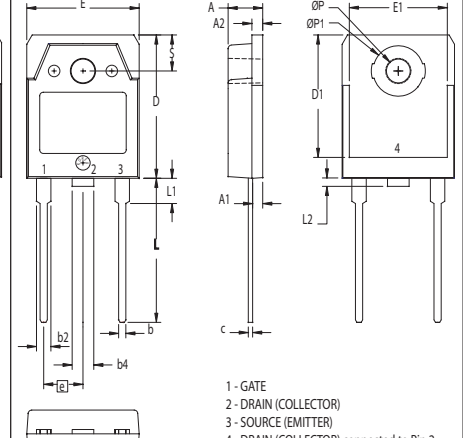
X017b TO-3P
