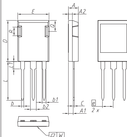
X016a ISOPLUS247
