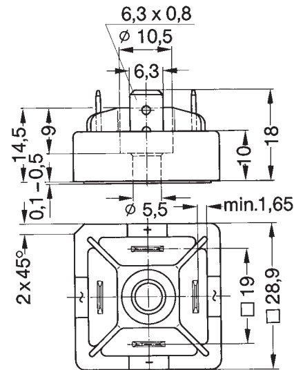
X115 FO-A
