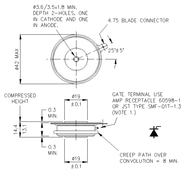
W8 - 101A212
