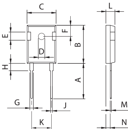
X014b TO-247 AD
