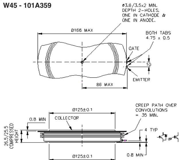
W45 - 101A359
