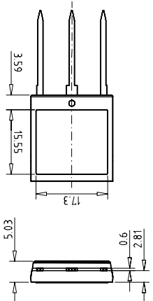
X024b ISOPLUS i4-Pac™
