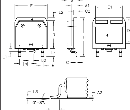
X019 TO-268 AA (D 3 PAK)
