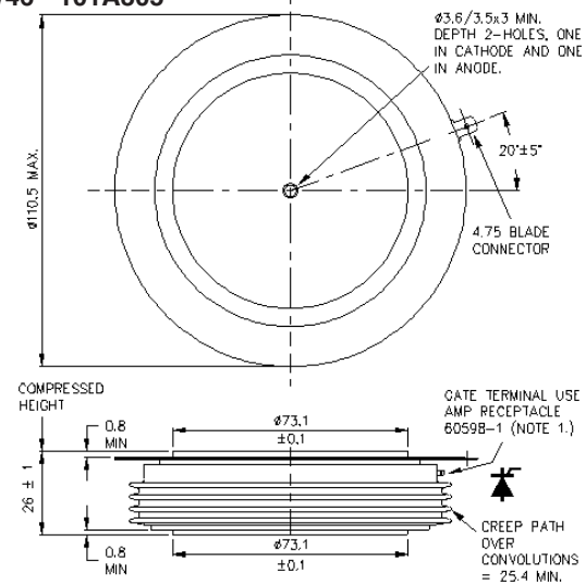
W46 - 101A305
