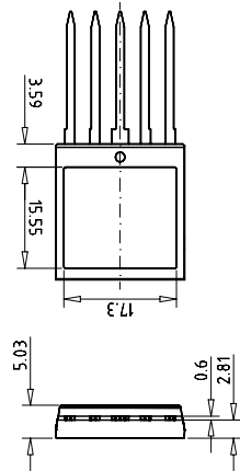
X024a ISOPLUS i4-Pac™
