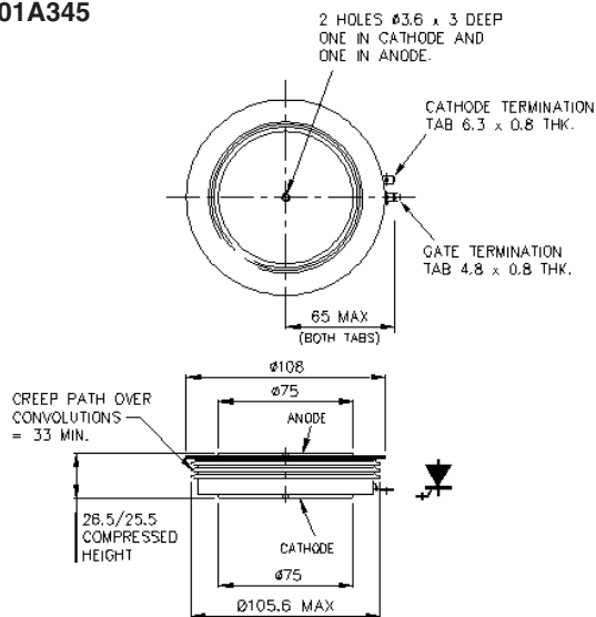
W32 - 101A345
