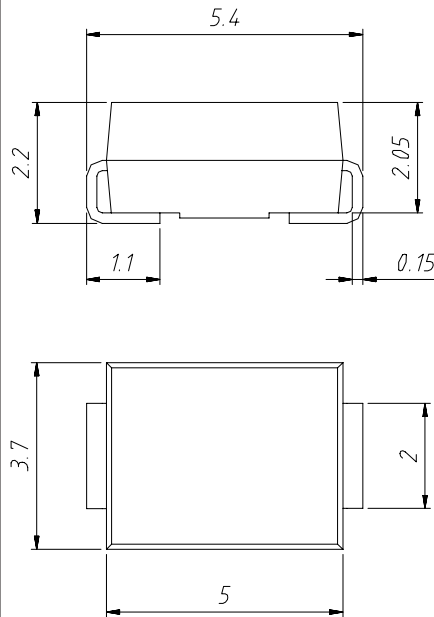
X002 SMB (DO-214 AA)
