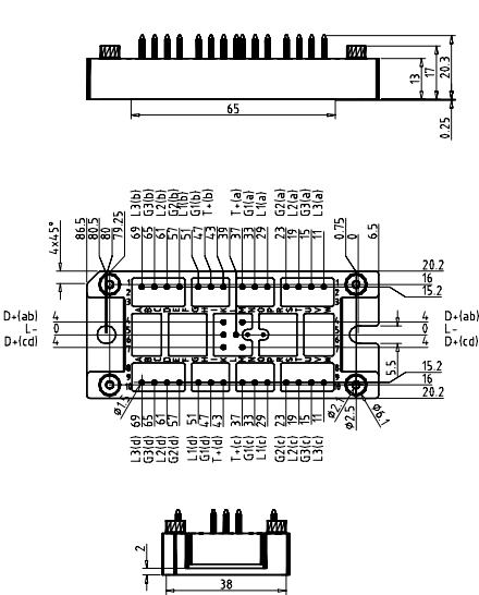
X104 V2-Pack
