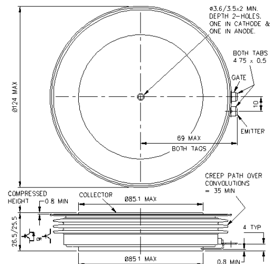
W44 - 101A340
