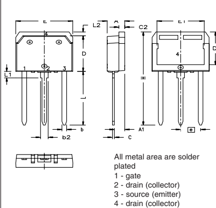
X018 TO-268 I 3 PAK
