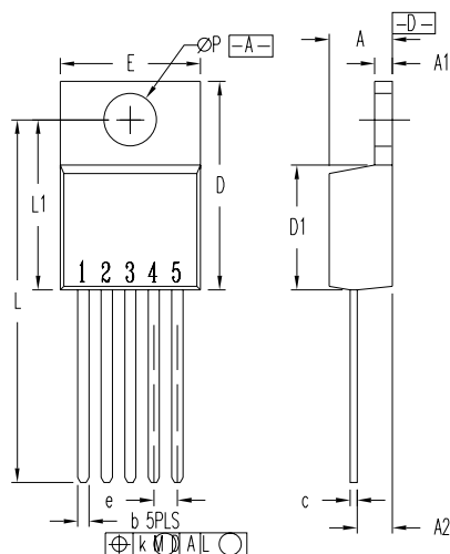
X006 TO-220 (5)
