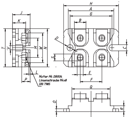
X028 ISOPLUS227™
