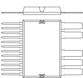
X026a ISOPLUS-DIL™ Weight = 25 g xxx-SL
