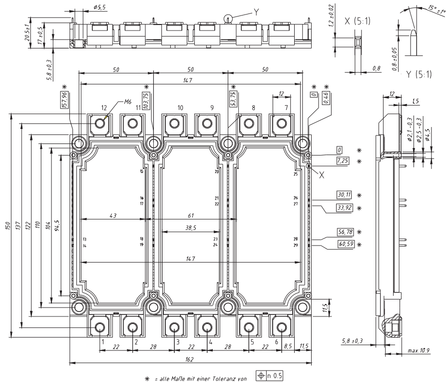
X116a FO-B-A
