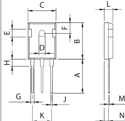
X014a TO-247 AD
