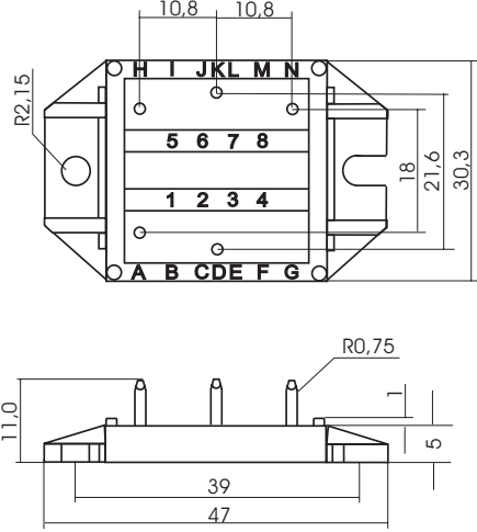
X100 Slim-PAC
