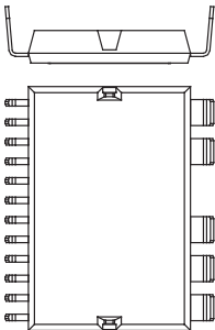
X026b ISOPLUS-DIL™ Weight = 25 g xxx-BL
