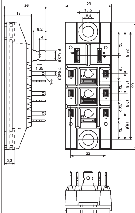
X118a FO-T-A
