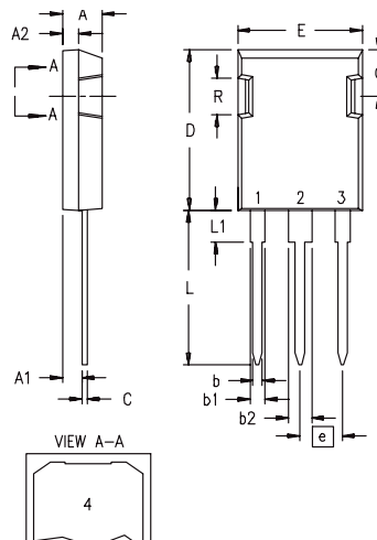
X015 PLUS247™
