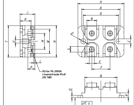
X027a SOT-227 B miniBLOC X027b SOT-227 UI miniBLOC
