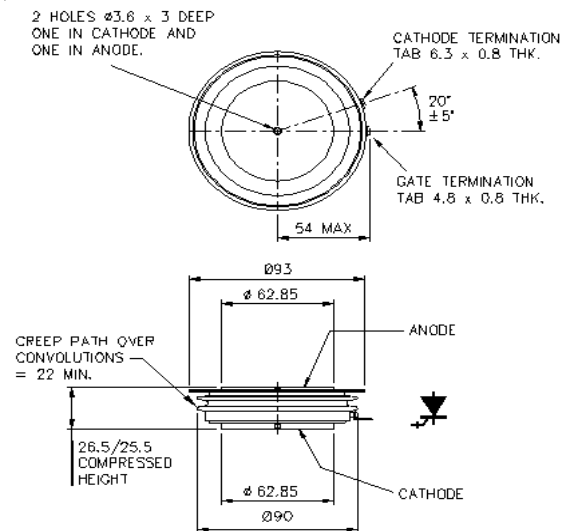
W31 - 101A344
