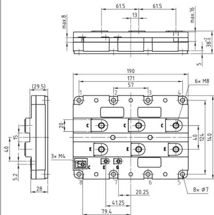
X134 E10-Pack
