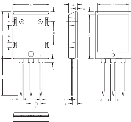
X022 ISOPLUS264
