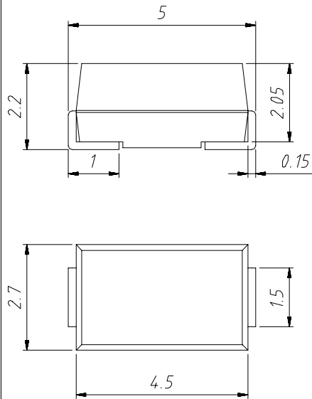
X001 SMA (DO-214 AC)
