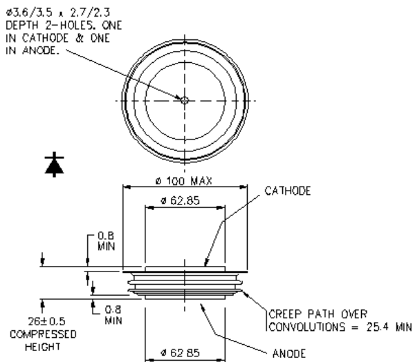
W43 - 100A320
