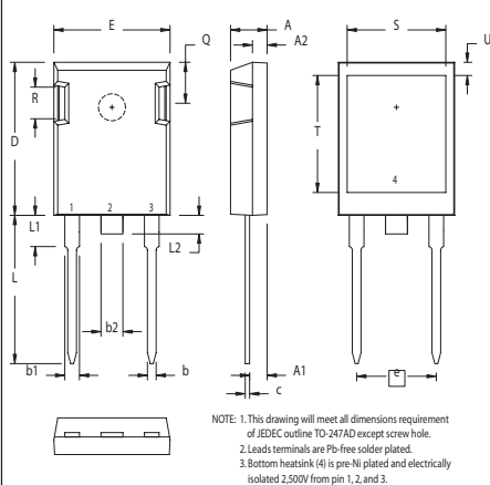
X016b ISOPLUS247
