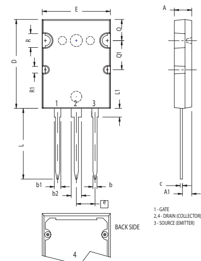
X021 PLUS264
